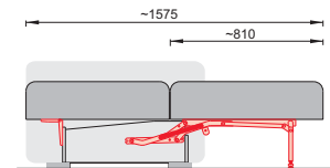
Fig. PF 075-A-5
