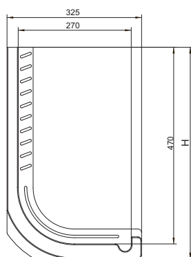
TP 004-5 H=510 ■ 0,62 ■ 10 TP 008-5 H=390 ■ 0,40 ■ 10 para/pair
