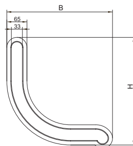
TP 001-4 H=308 B=234 ■ 0,10 ■ 50 TP 002-4 H=401 B=308 ■ 0,12 ■ 50 para/pair
